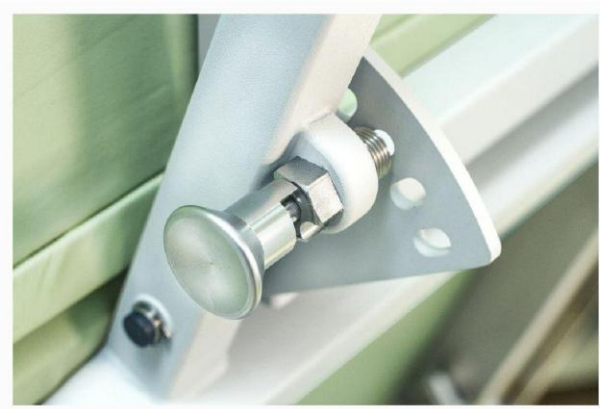
Fixare tetieră 0 – 40°
